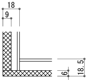
C部詳細
